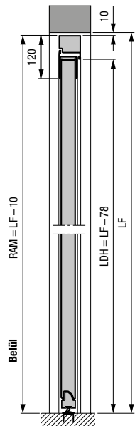
Mellékajtó alumínium blokkokkal, 2. profiltípus Beépítés a nyílásba
